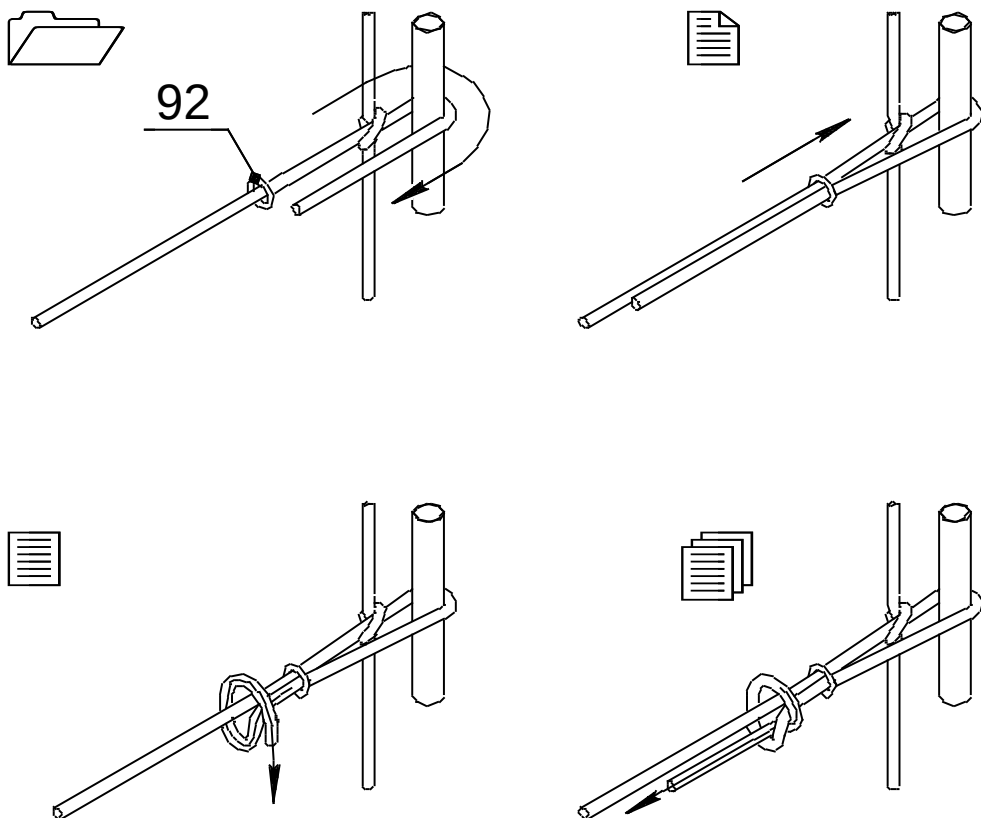
Рис.6 Схема крепления горизонтальных плетей сетки лаза
